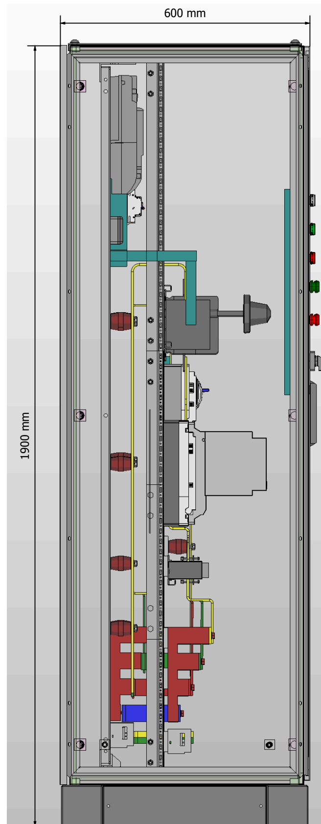
Вид слева
