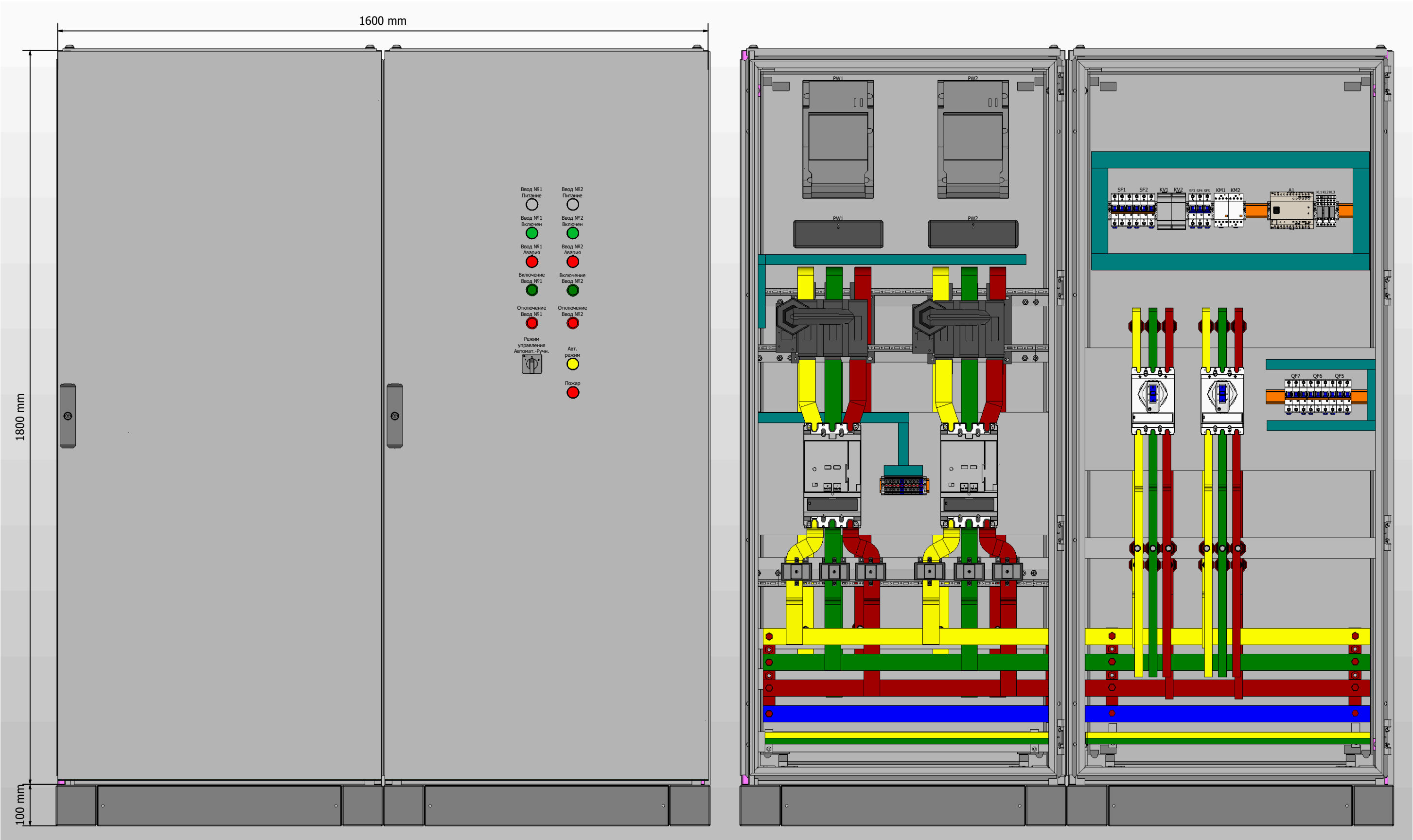
Вид спереди с дверями
